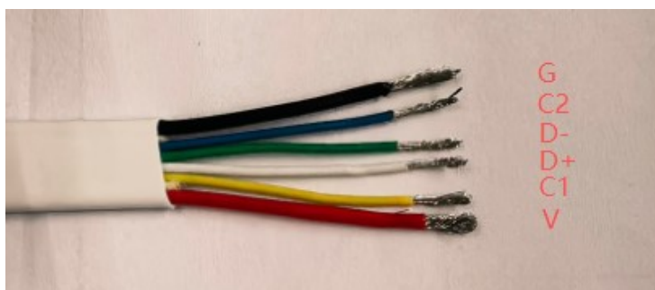
Rear wiring diagram 尾部接线示意图
